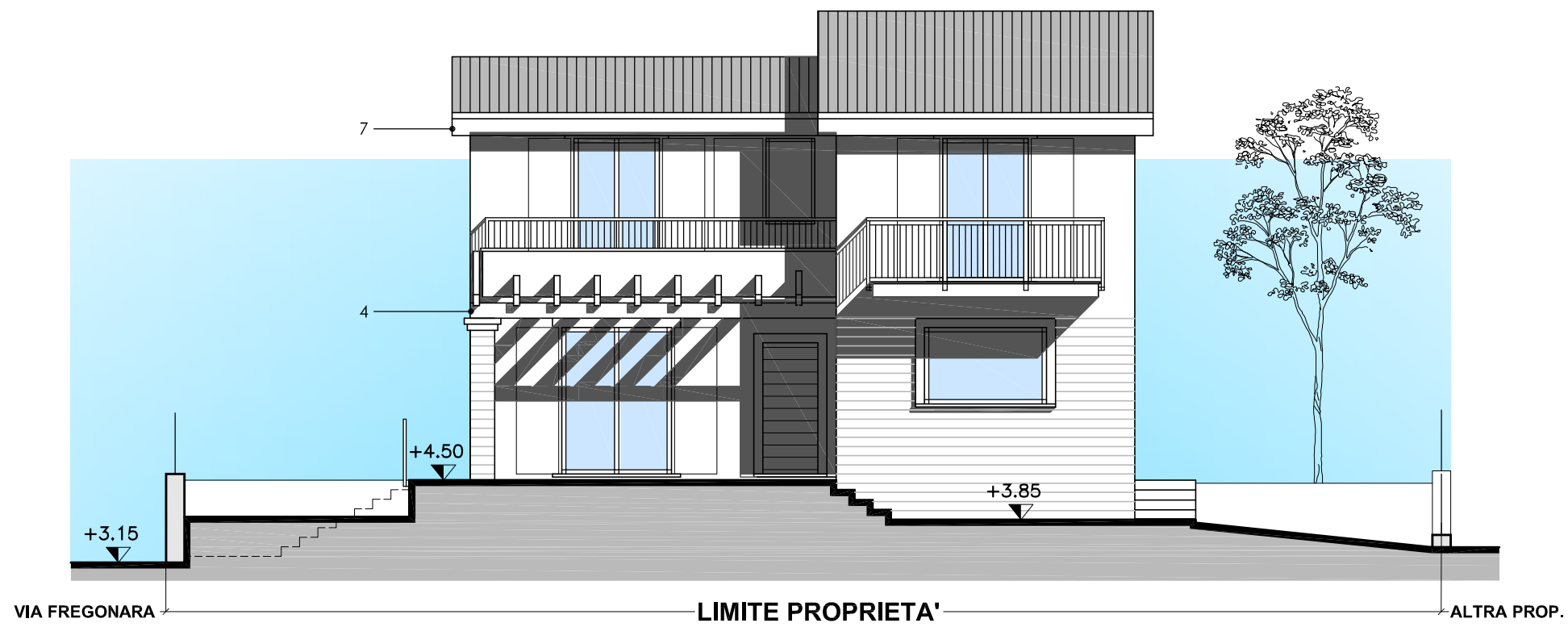
PROSPETTO EST_ Unità A
